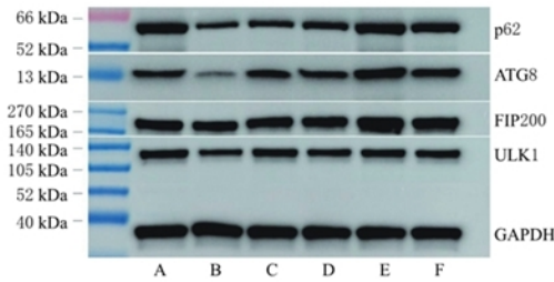
A:空白组;B:模型组;C:西药组;D:调中化湿汤低剂量组;E:调中化湿汤中剂量组;F:调中化湿汤高剂量组。
